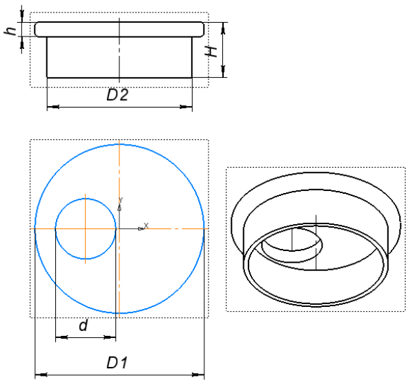
Рисунок 2.1- Модель заглушки с размерами
